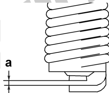
a) szczelina
